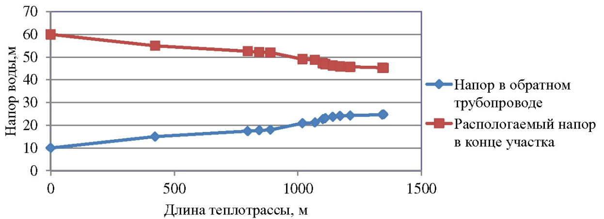
Рисунок 1-8. Пьезометрический график тепловой сети п. Элитный до здания ул. Лазурная, 38
