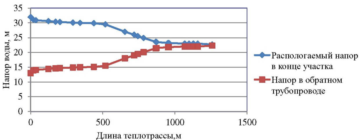
Рисунок 1-10. Пьезометрический график тепловой сети п. Мичуринский до здания ул. Ягодная, 52
