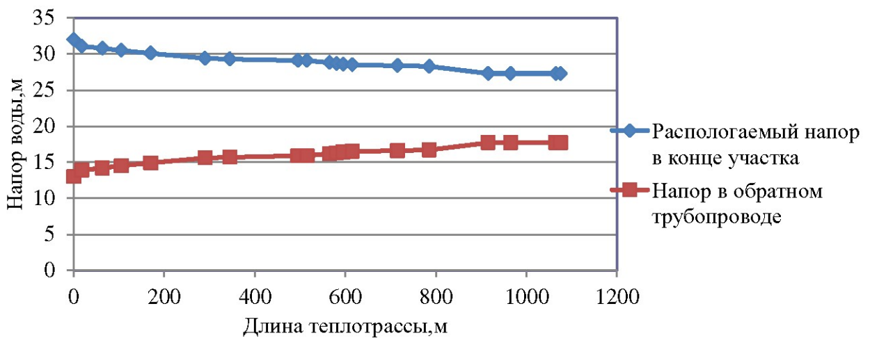
Рисунок 1-9. Пьезометрический график тепловой сети п. Мичуринский до здания ул. Снежная, 27
