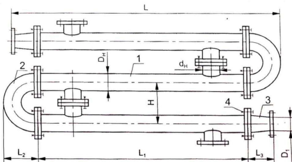
1 - секция разъемная типа РГ, 2 - калач соединительный, 3 - переход, 4 - крепеж
