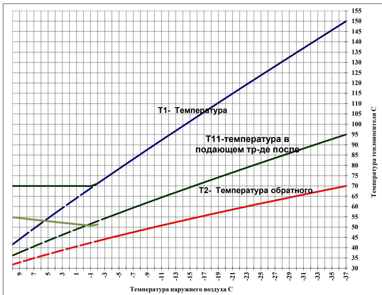
Рисунок 1-6. Температурный график
