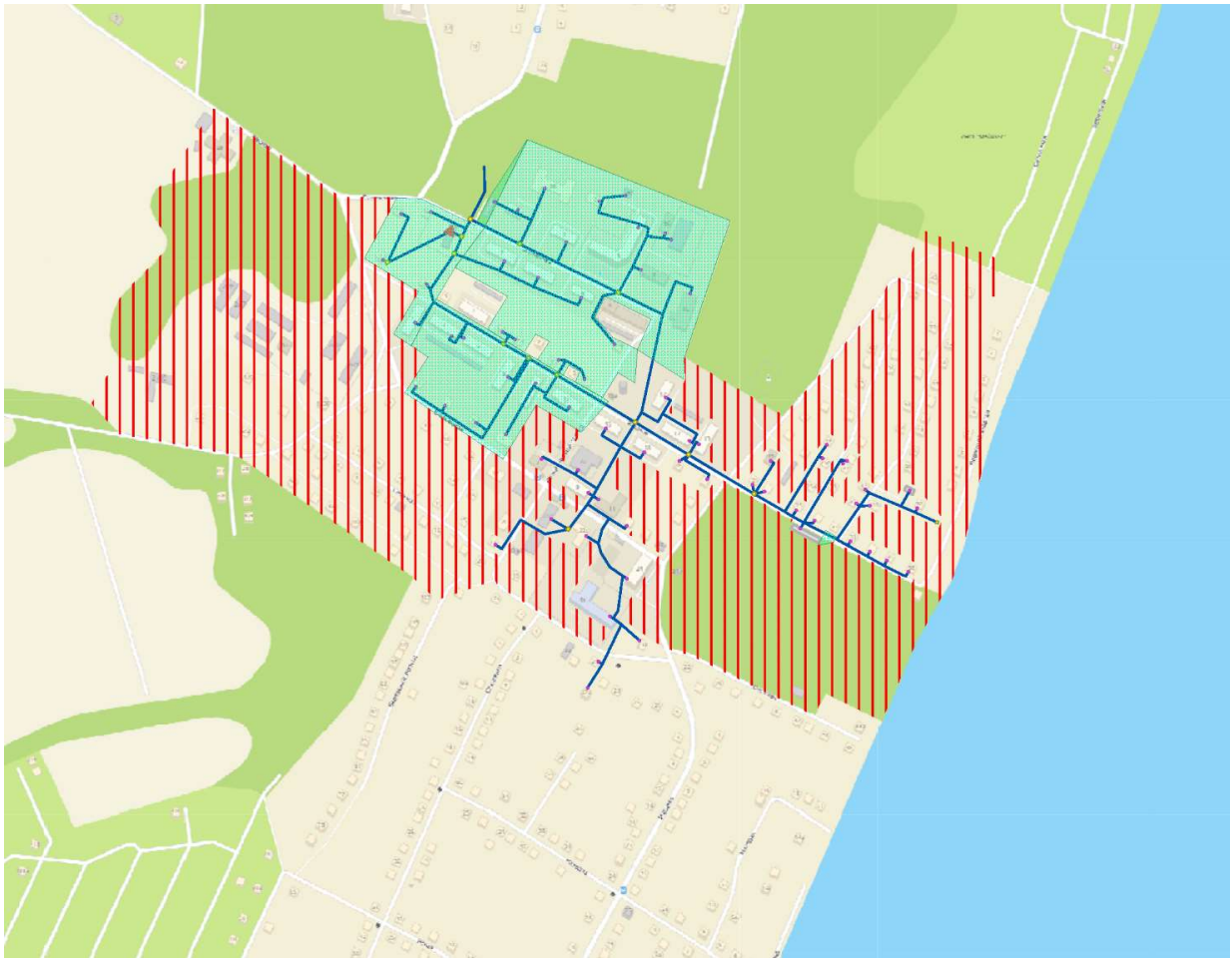
Рисунок 1-11. Зона действия централизованного теплоснабжения от ЦТП-9 п. Мичуринский
