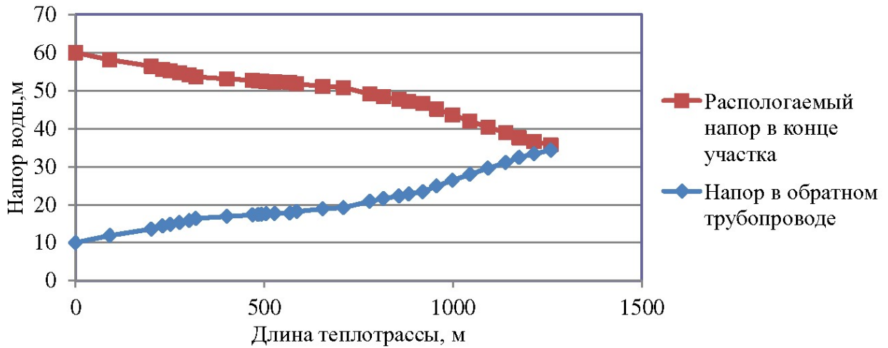
Рисунок 1-7. Пьезометрический график тепловой сети п. Элитный до здания ул. Полева, 4
