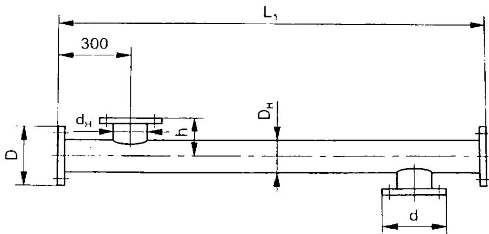
Рисунок 1-2. Секция разъемная типа РГ
