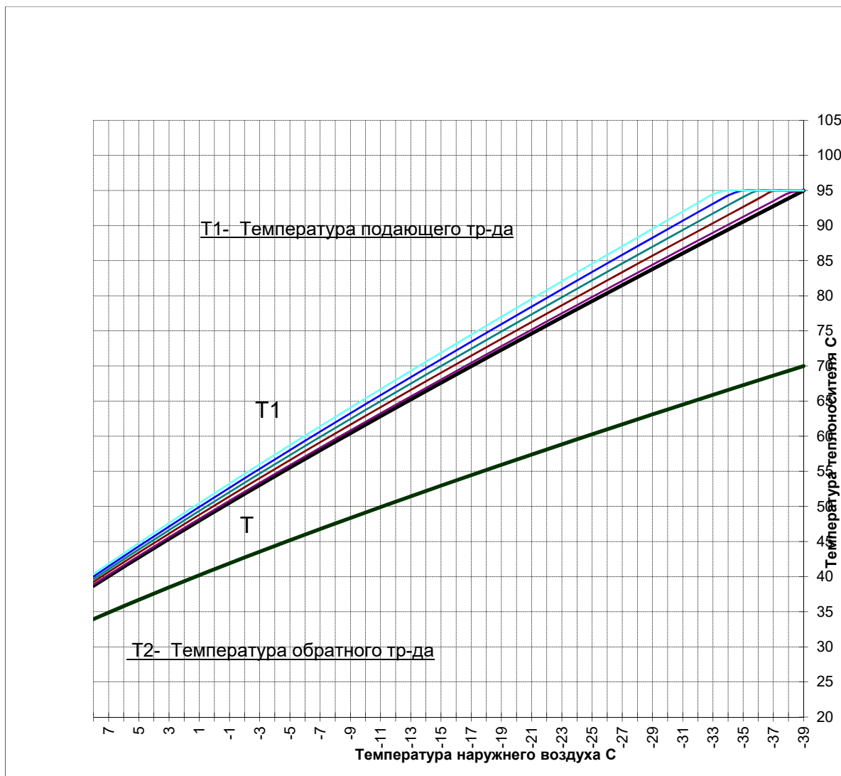
Рисунок 5-1. Температурный график ОО «Термооптима»
