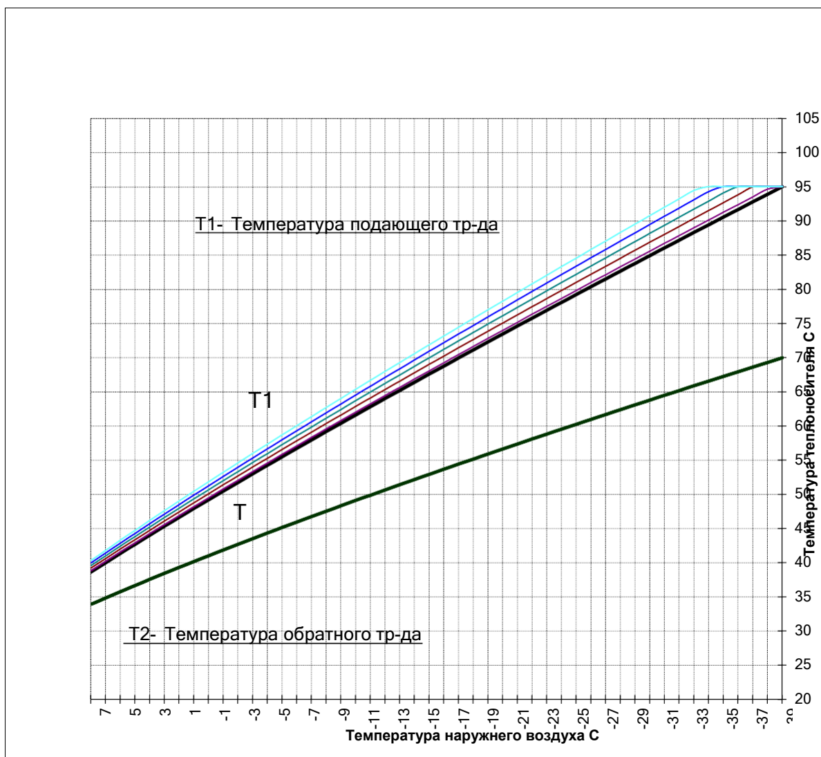
Рисунок 5-1. Температурный график ООО «Термооптима»
