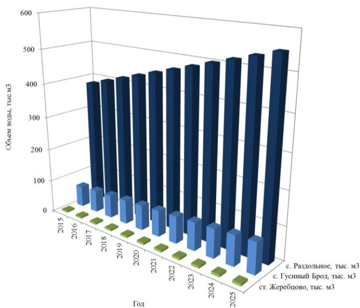
Рисунок 16 – Перспективный территориальный баланс водоснабжения
